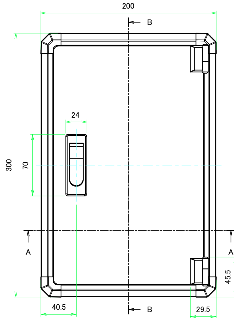
フレーム2側 / Frame2 side
