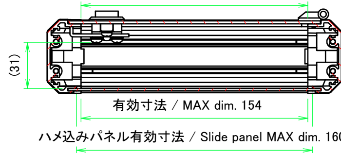
開閉パネル有効寸法 / Open-closing panel MAX dim. 154
