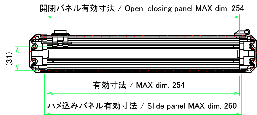
A-A (1:3)
