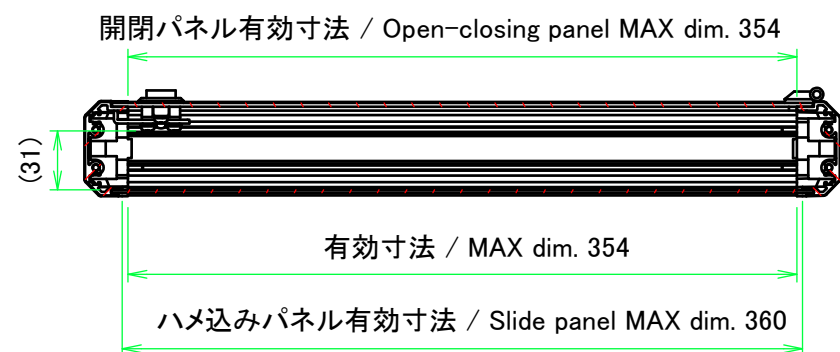
A-A (1:4)
