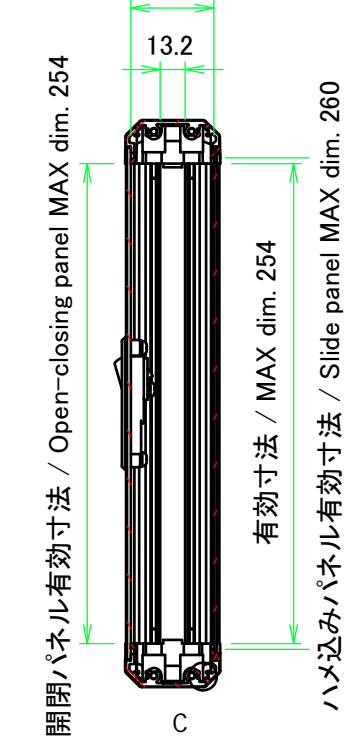
有効寸法 / MAX dim. 44
