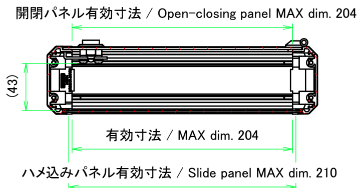
A-A (1:3.5)
