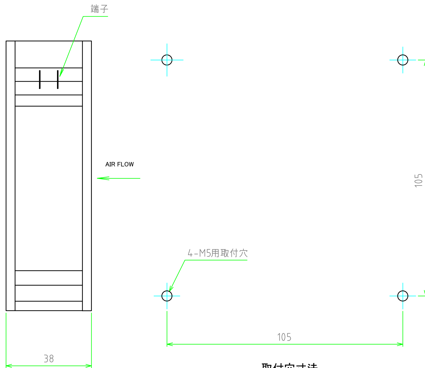
取付穴寸法
