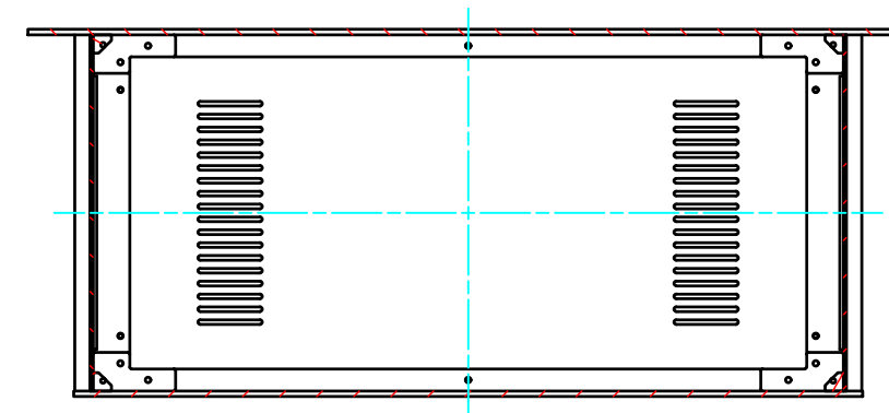
B-B (1 : 4.5)
