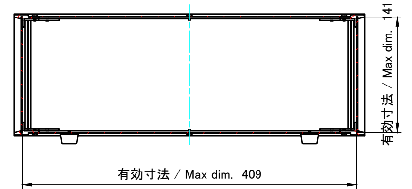
C-C (1 : 4.5)
