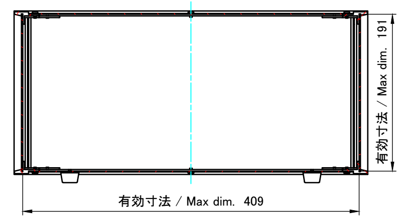
C-C (1 : 4.5)
