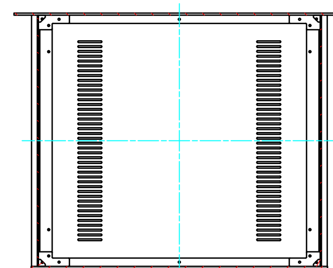
B-B ( 1 : 5.5 )
