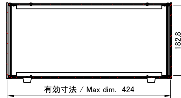
A-A (1:6)
