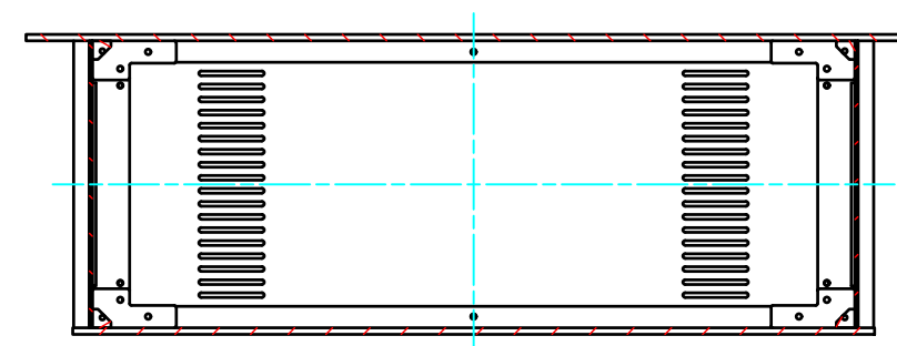
B-B (1 : 4.5)
