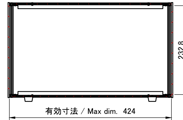
A-A (1:6)
