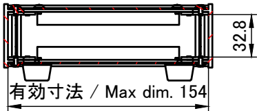
A-A ( 1 : 4 )
