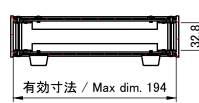
A-A (1 : 4.5)
