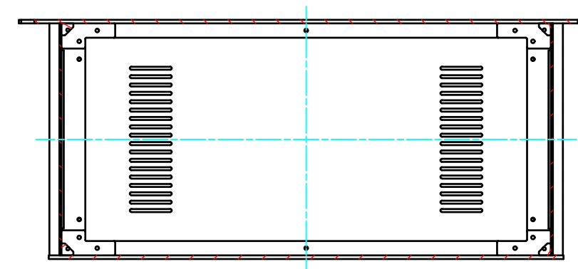
B-B (1 : 4.5)
