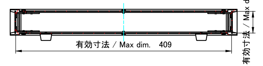
C-C ( 1 : 4.5 )
