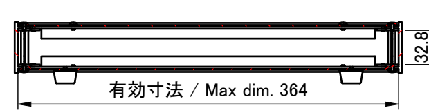
A-A (1:5)
