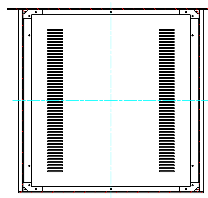
B-B ( 1 : 5.5 )
