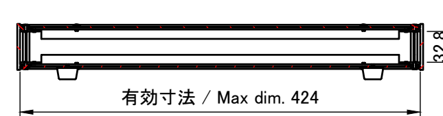
A-A ( 1 : 5.5 )
