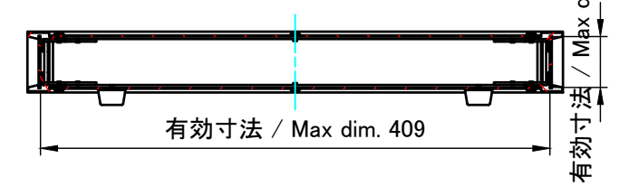
C-C ( 1 : 5.5 )
