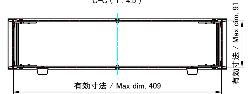
C-C ( 1 : 4.5 )
