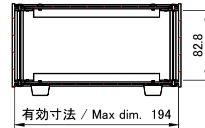
A-A ( 1 : 4.5 )
