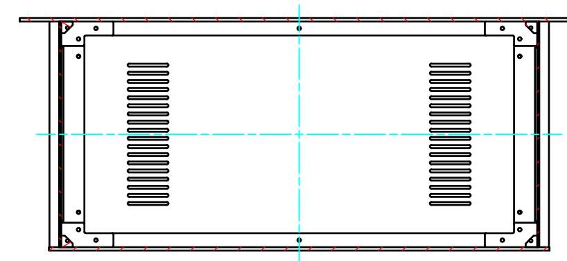
B-B ( 1 : 4.5 )
