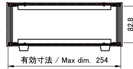
A-A (1:5)
