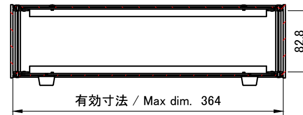
A-A (1:5)
