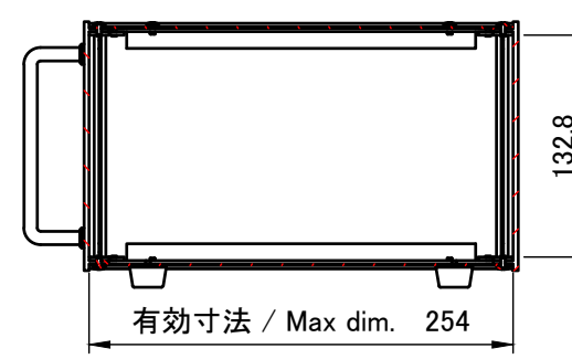
A-A (1:5)
