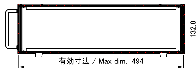
A-A (1:6.5)
