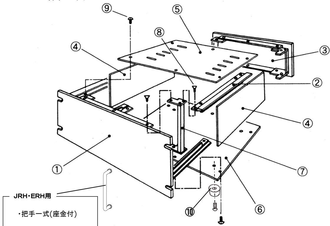
立体組立図
