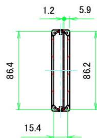
A-A (1:3)
