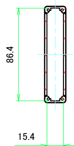
A-A (1:2.5)
