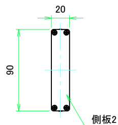
側板2
