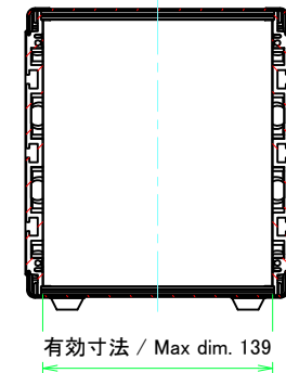
C-C ( 1 : 3.5 )
