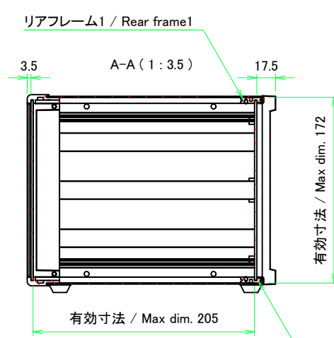
リアフレーム1 / Rear frame1
