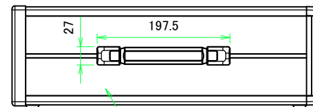
サイドフレーム2 / Side frame2
