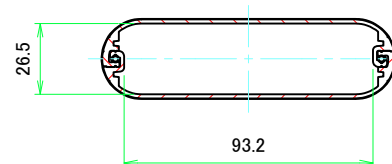
A-A (1:2)
