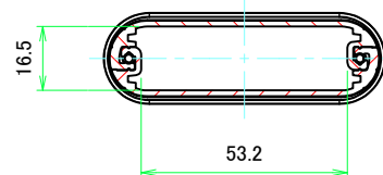
A-A (1:1.5)
