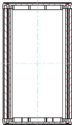
D-D (1:1.5)
