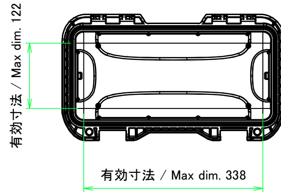
カバー 内視 / Cover Internal view
