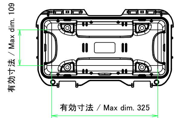
ベース 内視 / Base Internal view
