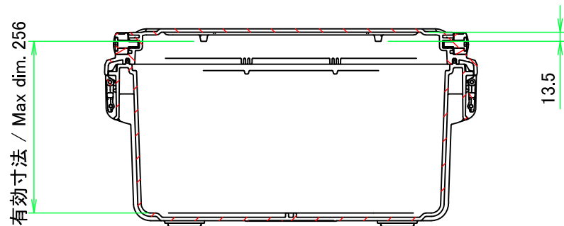
B-B ( 1:8 )
