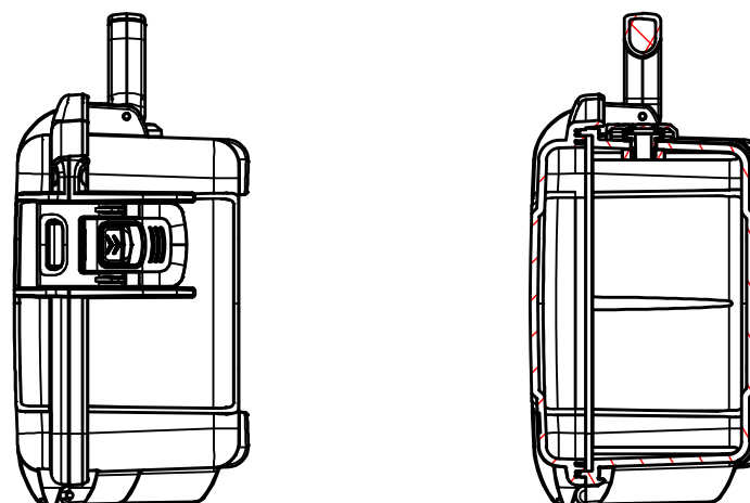
A-A (1:4)
