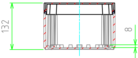
D-D
