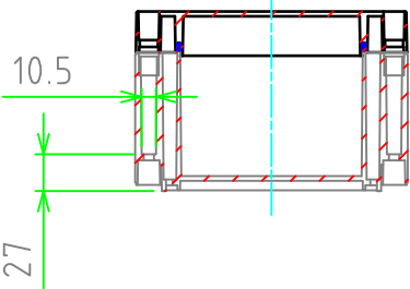
E-E
