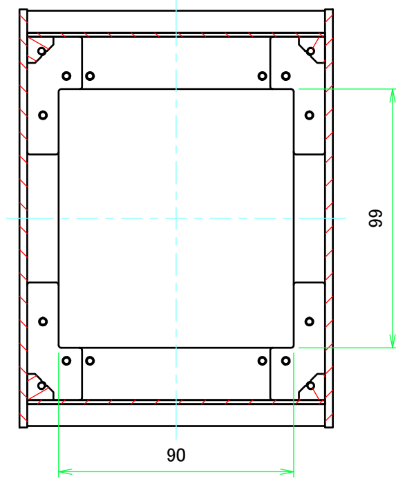
B-B (1:2)
