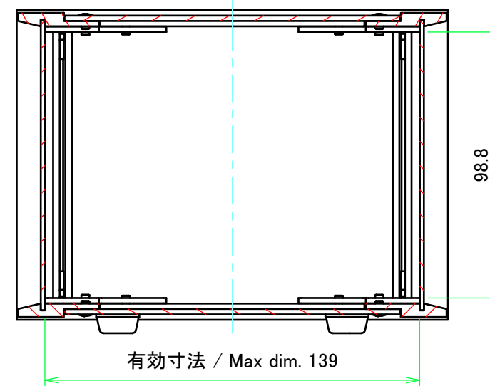
A-A (1:2)
