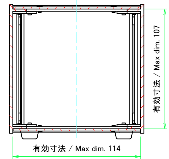
C-C (1:2)
