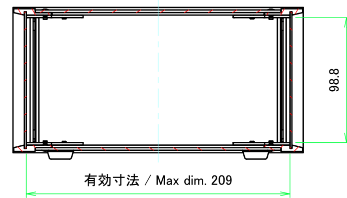
A-A ( 1 : 3 )
