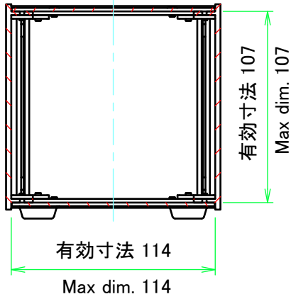
C-C ( 1 : 3 )
