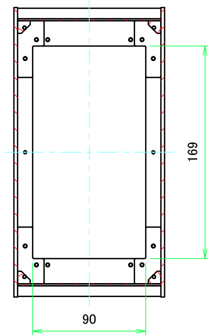
B-B ( 1 : 3 )
