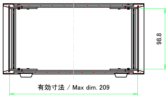
A-A ( 1 : 3 )
