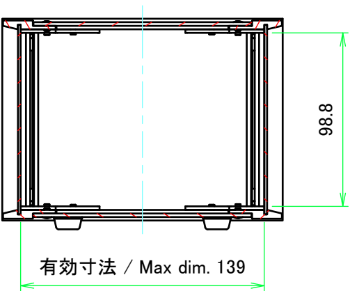
A-A ( 1 : 3 )
