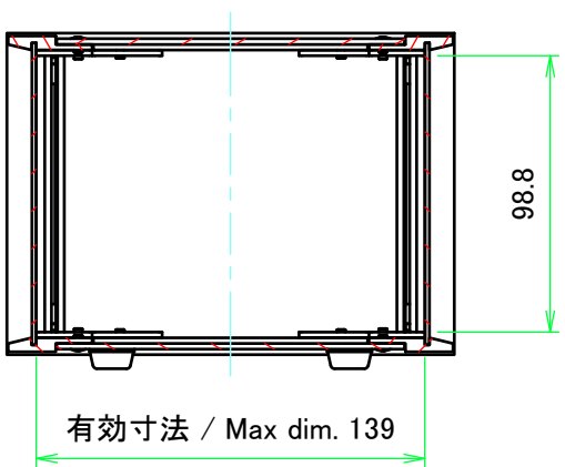
A-A ( 1 : 3 )
