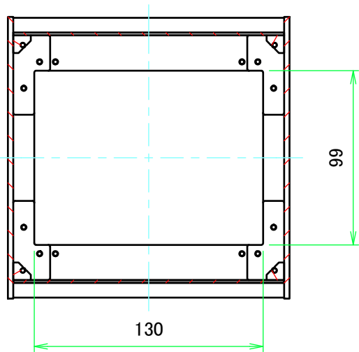
B-B ( 1 : 3 )
