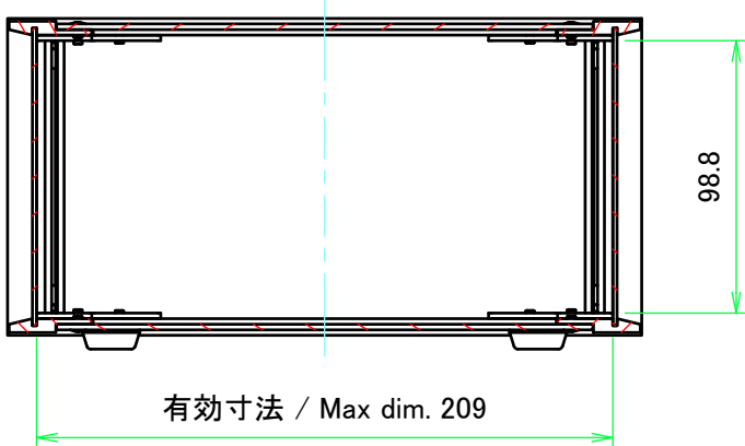
A-A ( 1 : 3 )
