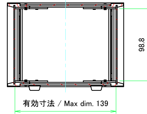
A-A (1:3)
