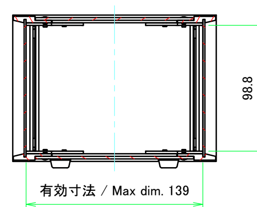
A-A (1:3)
