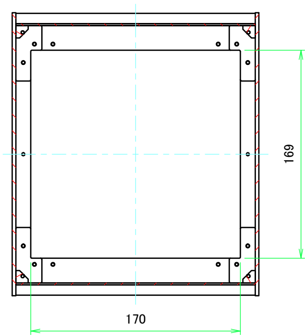
B-B ( 1 : 3 )
