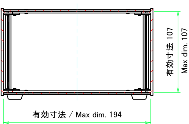
C-C ( 1 : 3 )
