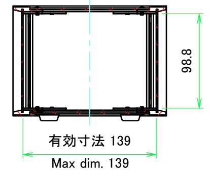
A-A ( 1 : 4 )
