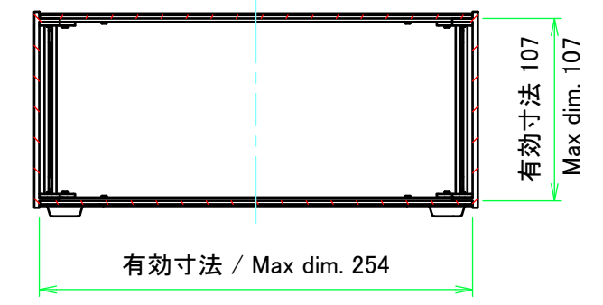
C-C ( 1 : 4 )
