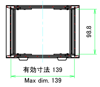
A-A ( 1 : 4 )
