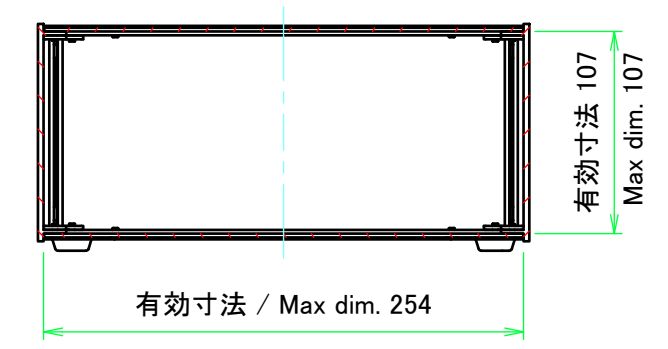
C-C ( 1 : 4 )
