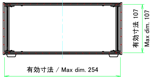
C-C ( 1 : 4 )
