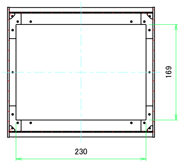
B-B ( 1 : 4 )
