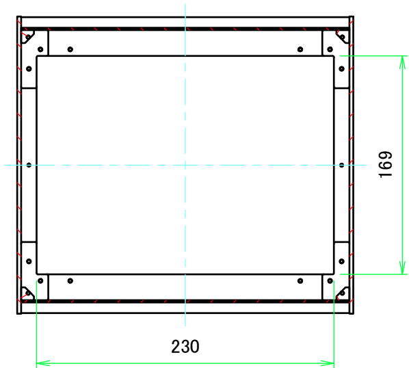
B-B ( 1 : 4 )
