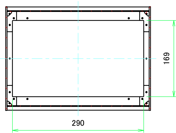
B-B ( 1 : 5 )
