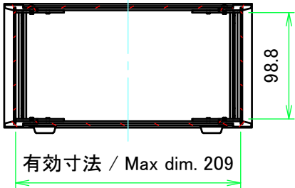
A-A ( 1 : 5 )
