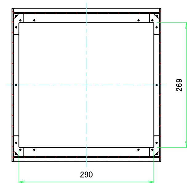
B-B ( 1 : 5 )
