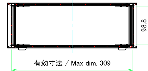
A-A ( 1 : 5 )
