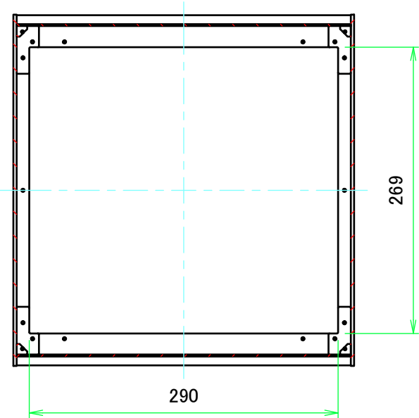
B-B ( 1 : 5 )
